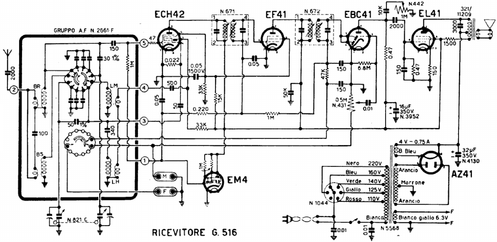
GELOSO - Mod. G 516. Onde medie da 190 a 580 m, quattro bande allargate ad onde corte, a 19, 25, 31 e 49 m. Media frequenza a 467 kc/s. Potenza di uscita 3 watt. Presa per magnetofono.
